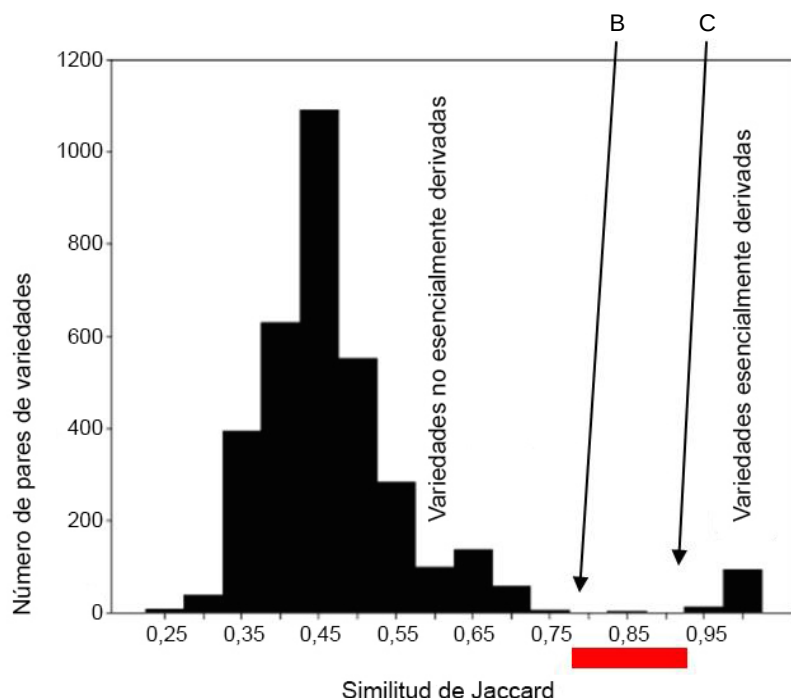
Figura 1. Gráfico extraído, a modo de ejemplo, del estudio de las variedades esencialmente derivadas de la rosa mediante la técnica de AFLP® (Vosman et al. , 2004). Distribución de las similitudes correspondientes a todos los pares de variedades. Todas las similitudes de las variedades esencialmente derivadas o mutantes tienen valores entre 0,95 y 1,0. Todas las variedades no esencialmente derivadas tienen valores de similitud menores que 0,80 y el 75%, menores que 0,50.
