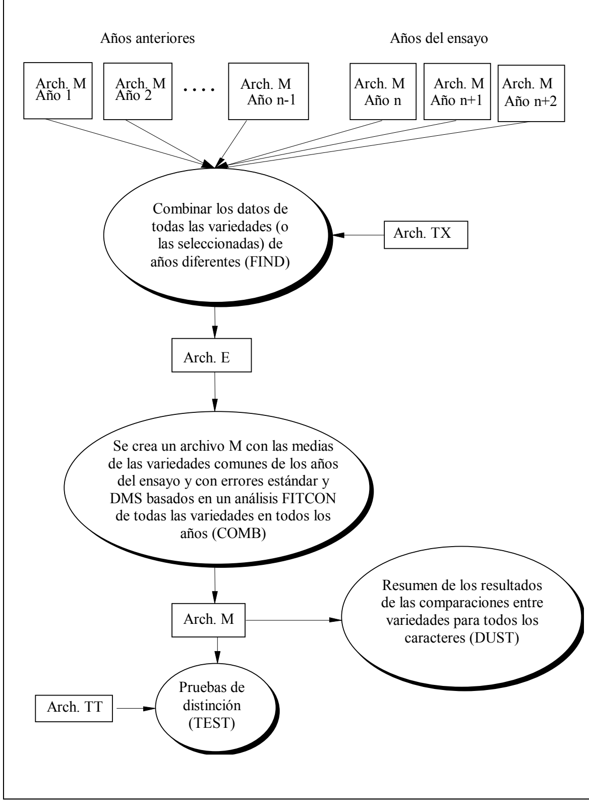
Figura B2. Flujograma de las etapas y módulos DUST utilizados para calcular las DMS de largo plazo y aplicar el COYD de largo plazo.
